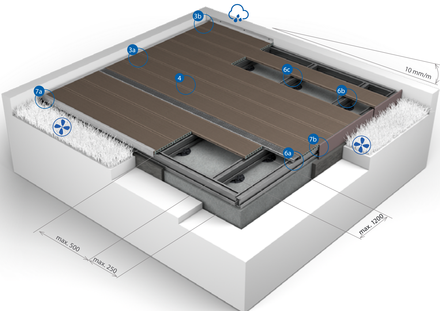
Example standard frame construction (over 19.5 cm construction height) Przykładowa standardowa konstrukcja ramy (wysokość konstrukcyjna powyżej 19,5 cm)
